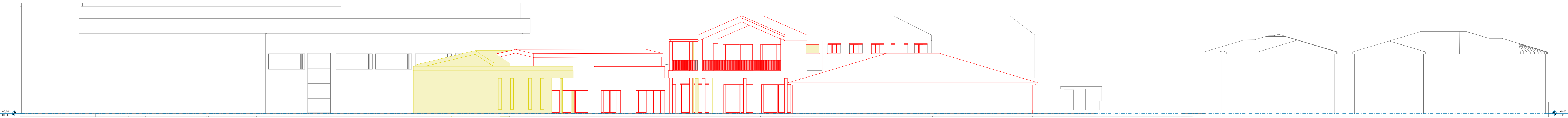
SEZIONE AMBIENTALE B-B - STATO COMPARATIVO - SCALA 1:200
